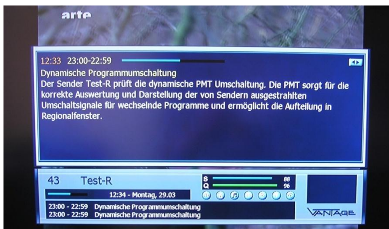
Abb2: „Test-R“: Testkanal auf Astra zur Überprüfung der dynamischen PMT-Umschaltung von Digiteempfängern
